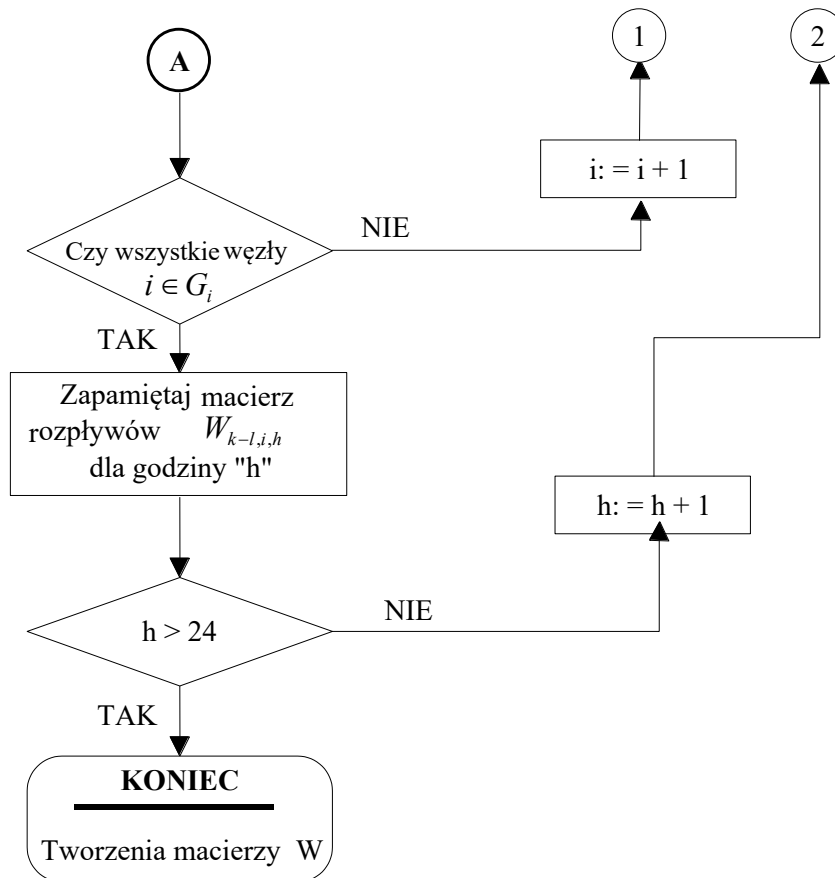
Rys. Z.3. Algorytm tworzenia macierzy rozpływów W
