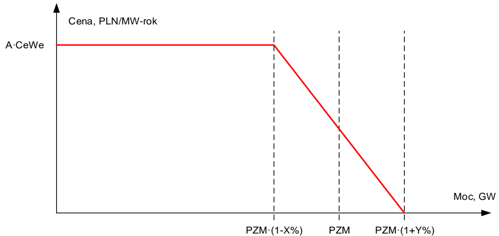
Rys. 8.2.1.1– Krzywa zapotrzebowania na moc (rysunek poglądowy)
