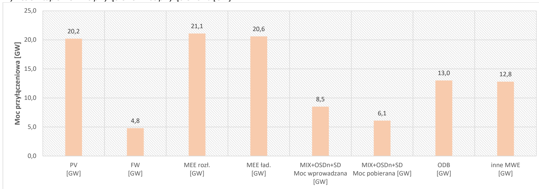
Wykres 3. Etap UMOWY o przyłączenie - moc przyłączeniowa [GW].
