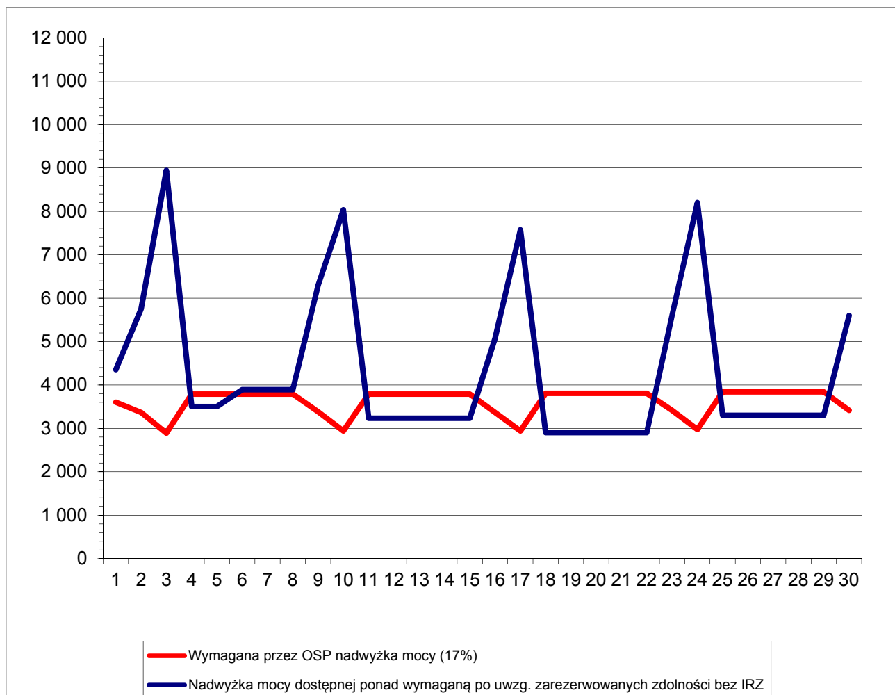
Rys.1 Wartości nadwyżki mocy dostępnej dla OSP dla poszczególnych dób w czerwcu 2018
