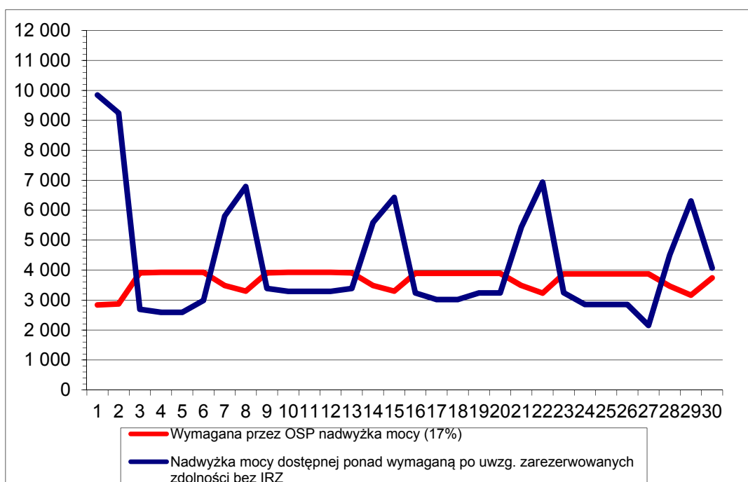
Rys.1 Wartości nadwyżki mocy dostępnej dla OSP dla poszczególnych dób w kwietniu 2018
