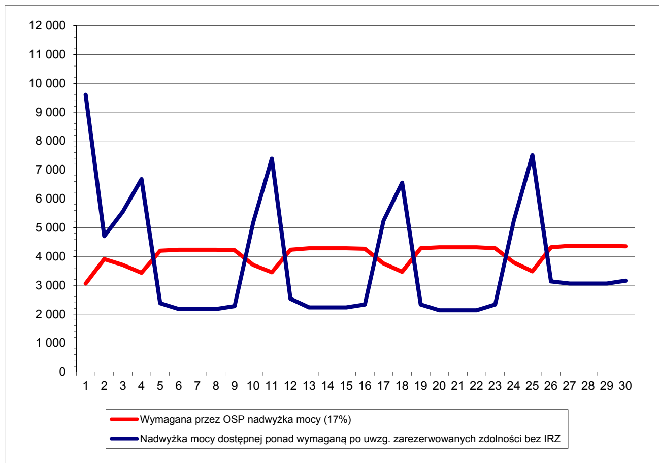
Rys.1 Wartości nadwyżki mocy dostępnej dla OSP dla poszczególnych dób w listopadzie 2018 r.
