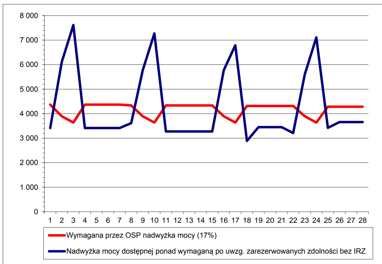
Rys.1 Wartości nadwyżki mocy dostępnej dla OSP dla poszczególnych dób w lutym 2019 r.
