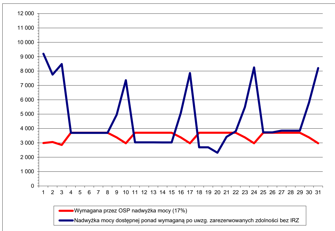
Rys.1 Wartości nadwyżki mocy dostępnej dla OSP dla poszczególnych dób w maju 2020 r.
