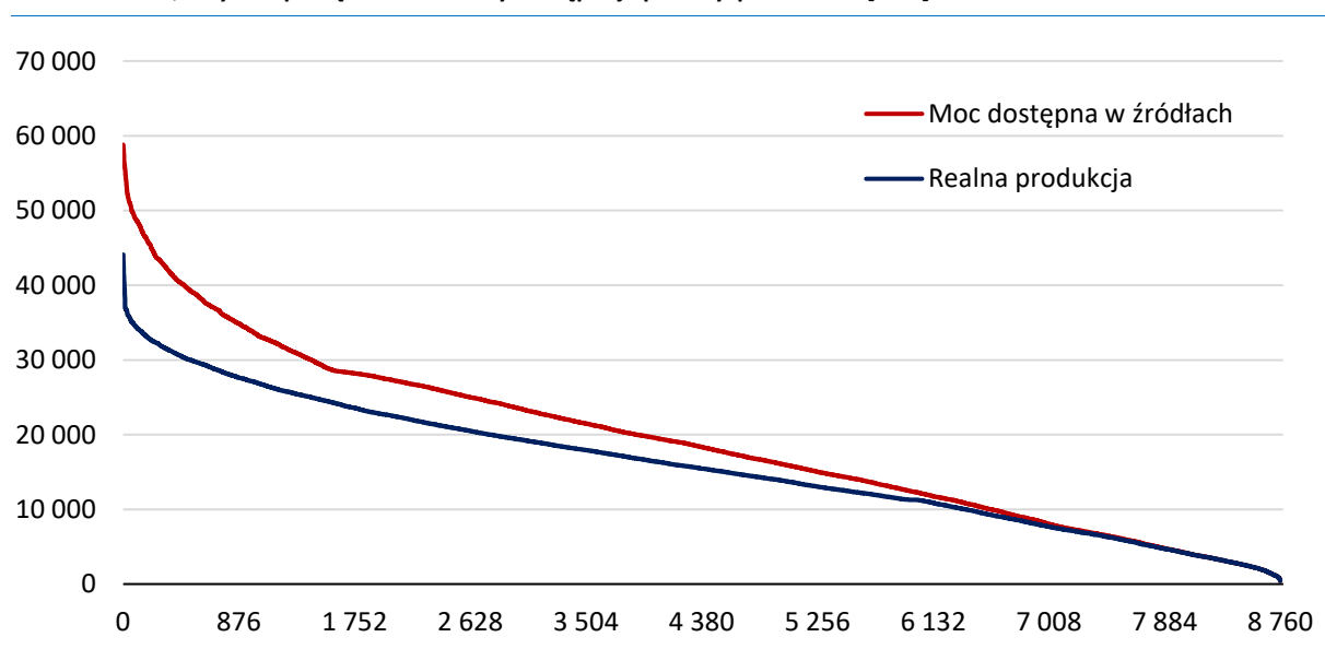
Rys. 4-11 Rzeczywista moc generacji ze źródeł fotowoltaicznych, lądowych i morskich elektrowni wiatrowych oraz moc dostępna, wynikająca z energii pierwotnej, w scenariuszu SDT, w roku 2034 i roku klimatycznym SWS
