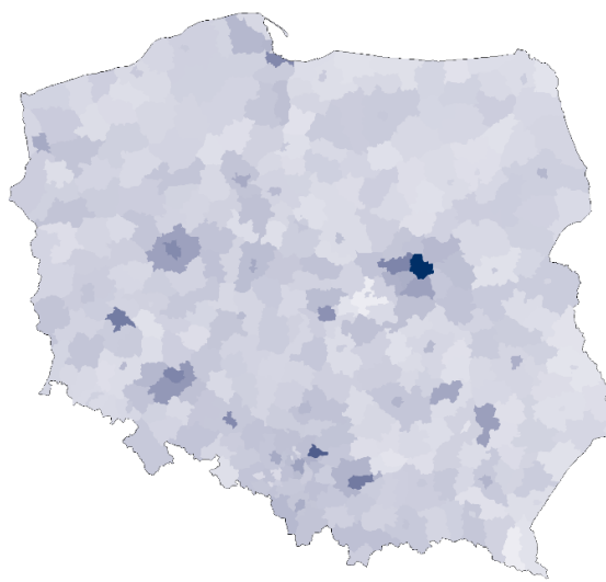
Rys. 4-5 Rozkład zapotrzebowania na moc elektryczną w szczycie zimowym w roku 2034 – scenariusz SDT
