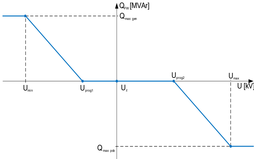
Rysunek 3.3.4.2. 1. Charakterystyka statyczna regulacji napięcia PPM przyłączonego do sieci WN lub NN gdzie:
