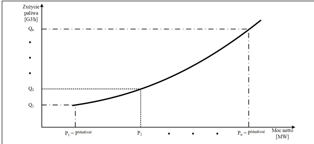
Rysunek 14.1. Charakterystyka zużycia energii chemicznej w paliwie w funkcji generowanej mocy elektrycznej netto.
