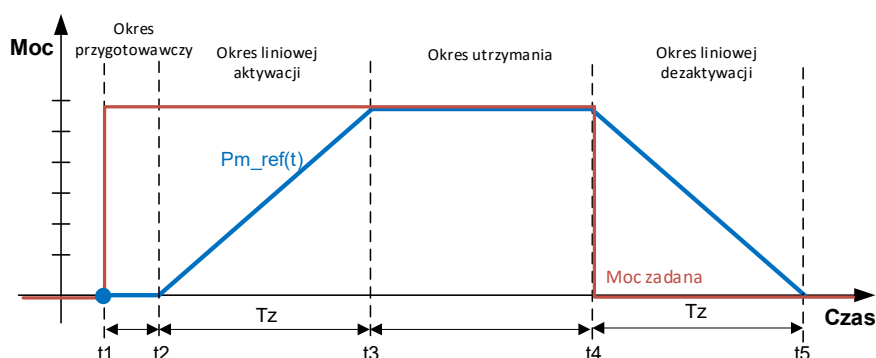
Rysunek 3.6.4.2. 1. Charakterystyka realizacji mocy zadanej w torze mFRRd
