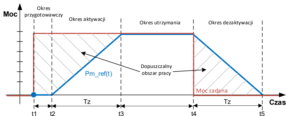
Rysunek 3.6.4.3. 1. Charakterystyka realizacji mocy zadanej w torze mFRRn
