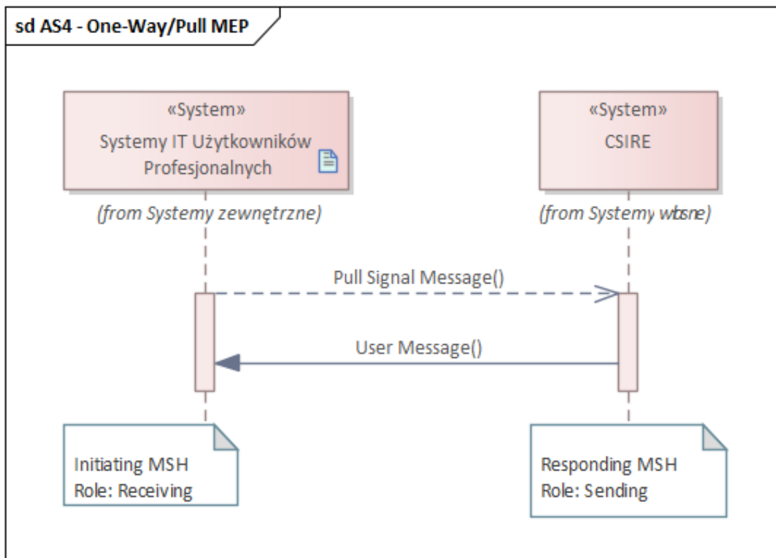
Rysunek 6 One-Way/Pull MEP
