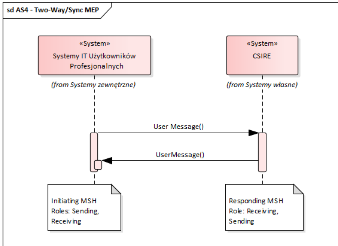
Rysunek 55 Two-Way/Sync MEP
