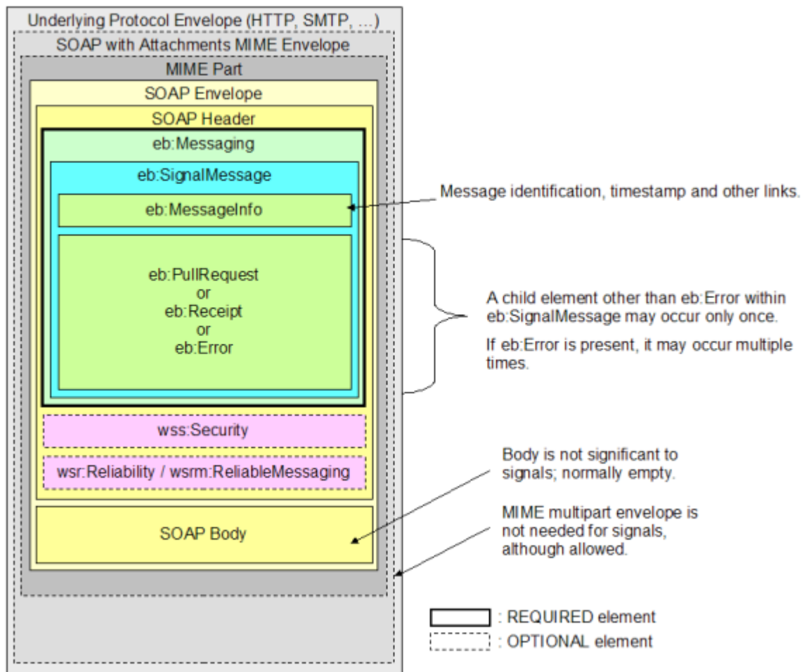
Rysunek 22 Struktura wiadomości sygnałowej (Signal Message Structure, [ebMS3CORE])
