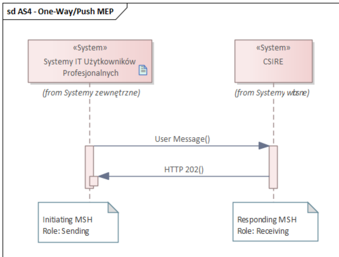
Rysunek 33 One-Way/Push MEP
